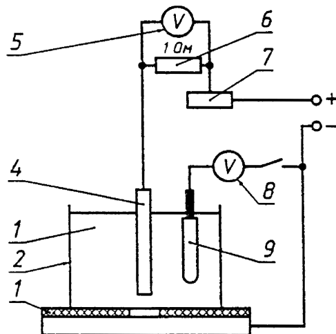
Рисунок В.3 - Схема проведения испытания образцов покрытий на пластинах (картах) для определения площади отслаивания с применением магниевого анода
