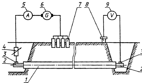
1 - трубопровод; 2 - неизолированный конец трубопровода; 3 - контакты; 4 - резистор; 5 - амперметр; 6 - источник постоянного тока; 7 - временное анодное заземление; 8 - медно-сульфатный электрод сравнения; 9 - вольтметр
